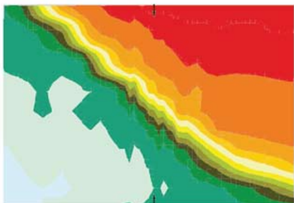
Praėjimas be oro užuolaidos
